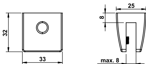
Размеры светильника:
