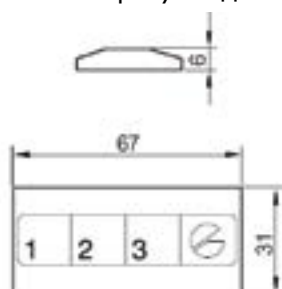
Размеры пульта ДУ:
