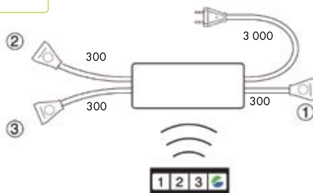
Схема и размеры выключателя:
