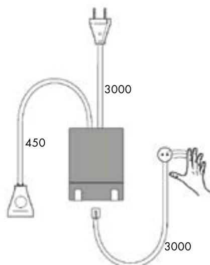
Схема и размеры выключателя:
