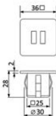
Размеры розетки:
