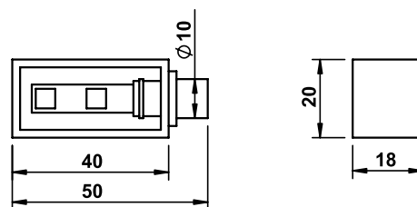
Размеры светильника:
