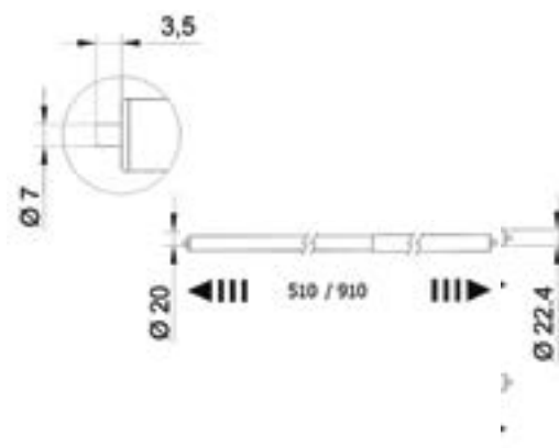
Размеры штанги:
