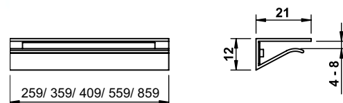
Размеры светильника:
