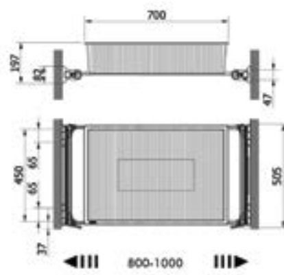
Размеры ящика:
