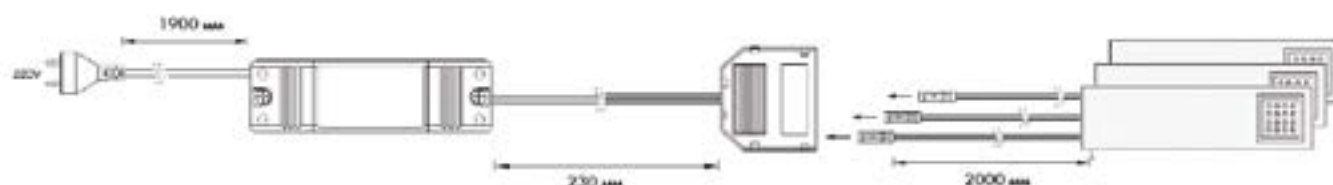
Подключение светильников к трансформатору:
