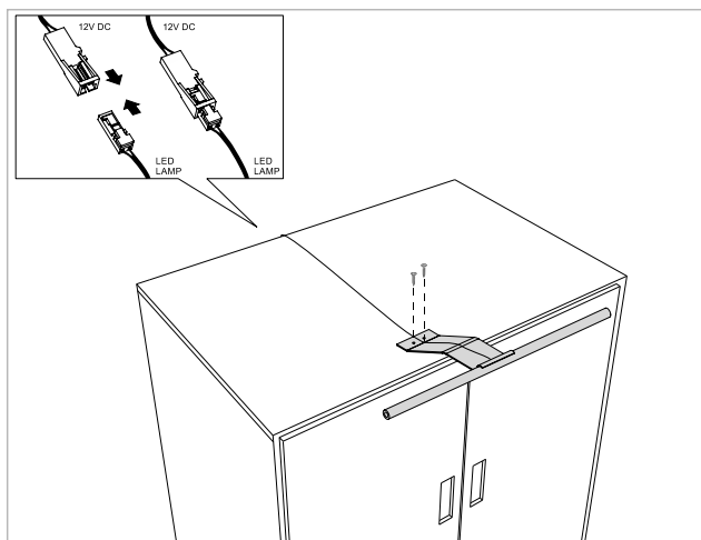
Схема крепления светильника:
