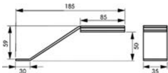
Размеры светильника:
