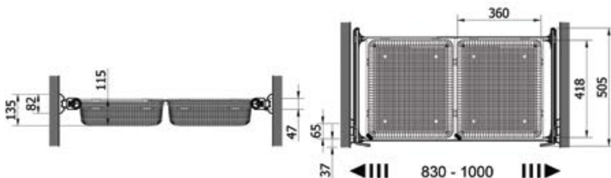
Размеры корзин:
