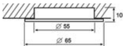
Схема врезного светильника:
