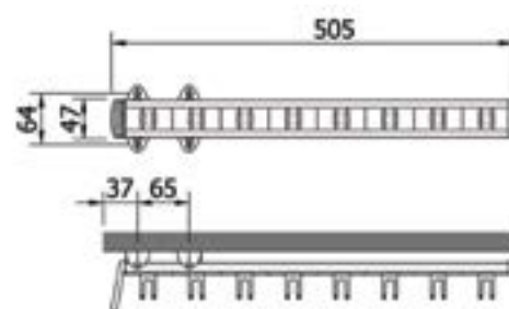
Размер держателя:
