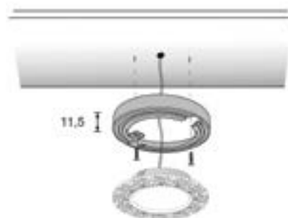
Схема накладного кольца:
