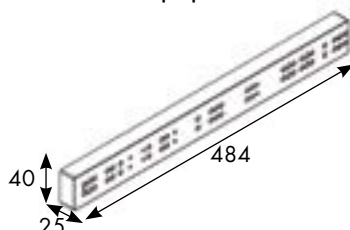
Размер проставки:
