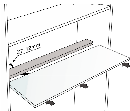
Схема крепления светильника:
