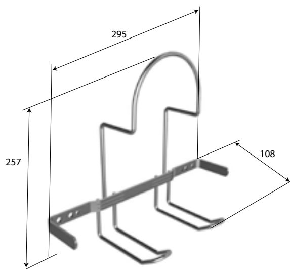
Размер держателя:
