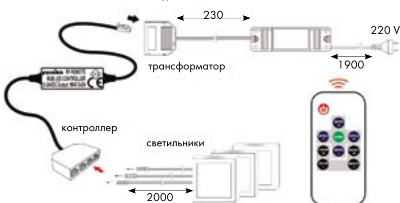
Схема подключения светильников:
