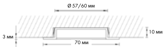
Размеры светильника:
