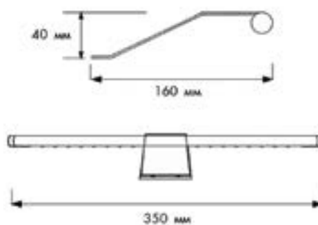
Размеры светильника:
