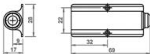
Размеры выключателя:
