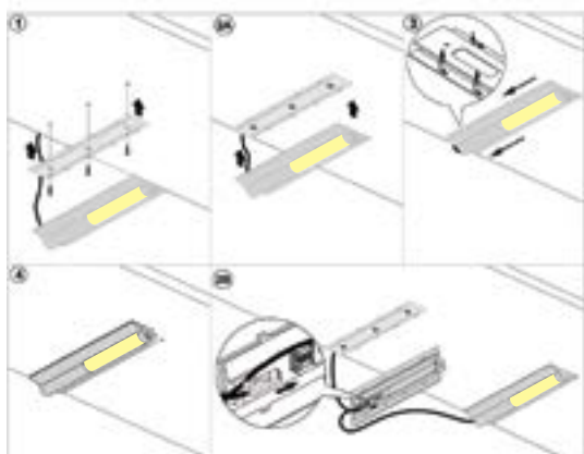
Схема крепления светильника:
