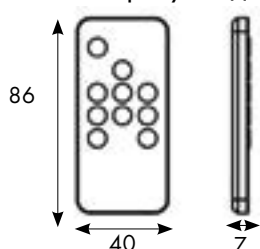
Размеры пульта ДУ:
