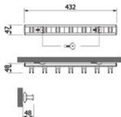
Размер держателя:
