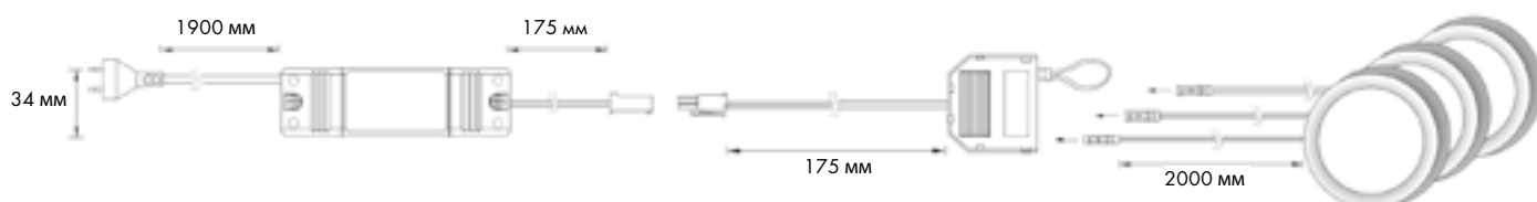
Подключение светильников к трансформатору:
