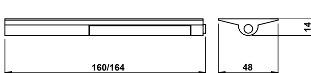
Размеры светильника:
