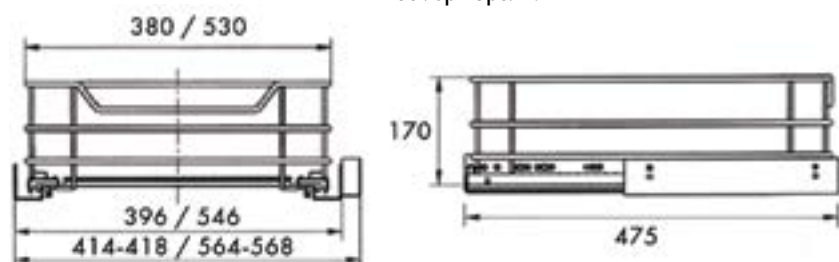
Размер корзин:
