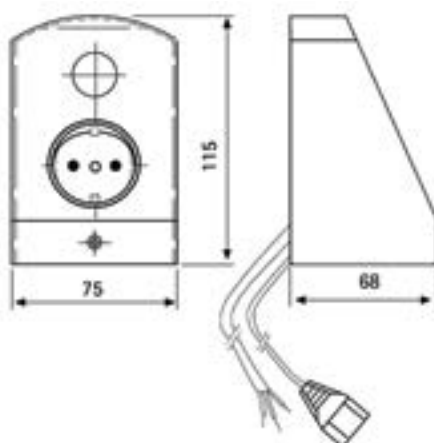
Размеры блока:
