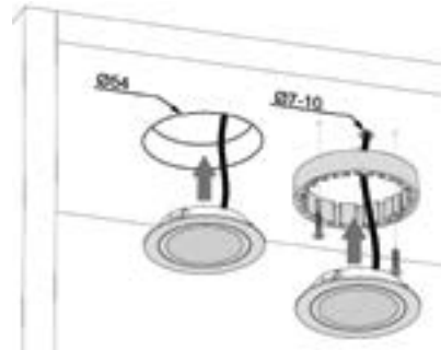
Схема установки светильника:
