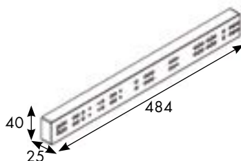
Размер проставки:
