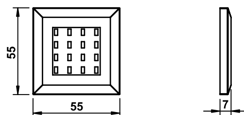
Размеры светильника:
