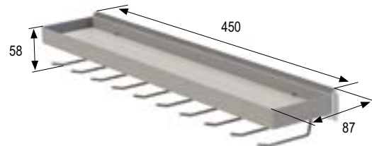
Размер держателя:
