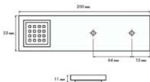
Размеры светильника:
