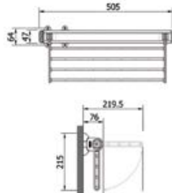
Размер держателя:
