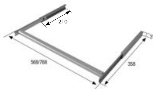
Размеры штанги:
