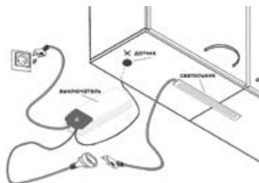
Установка выключателя:
