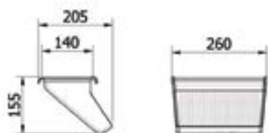
Размер лотка:
