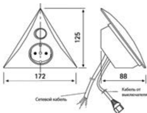
Размеры блока:
