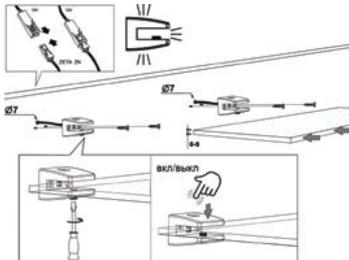
Установка светильника:
