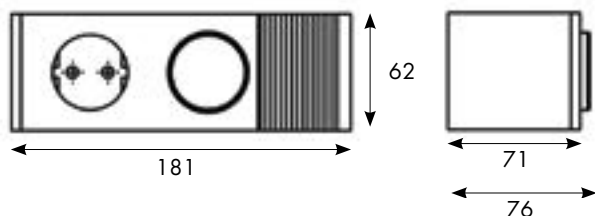
Размеры блока:
