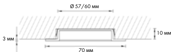
Размеры светильника:
